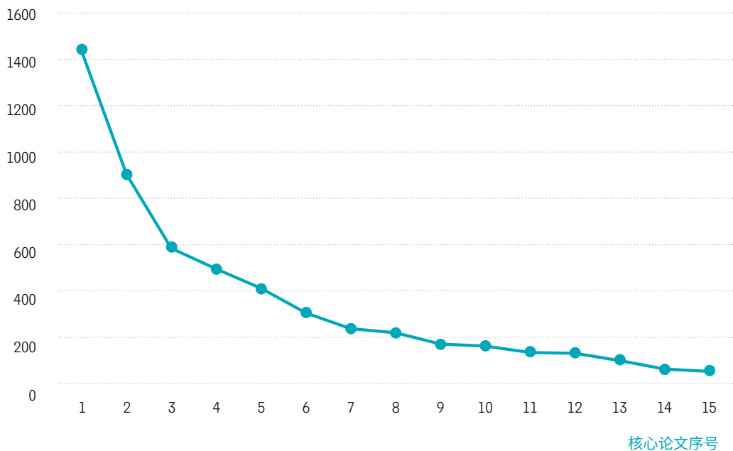
图 18 “高效金属卤化物钙钛矿发光二极管”研究前沿中核心论文的被引频次分布曲线
