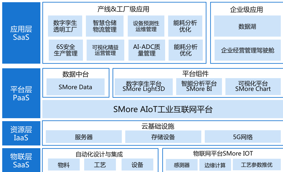
思谋SMore AIoT工业互联网平台系统架构
